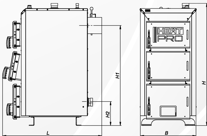
Рисунок 1 – Позначення габаритів котла
