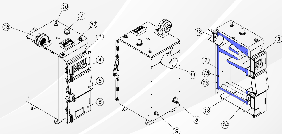
Зовнішній вигляд котла
